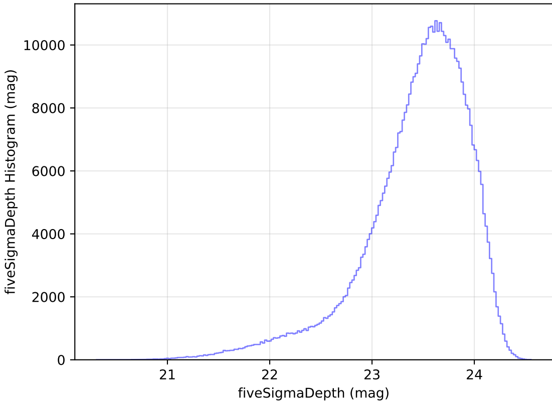
weather_cloudso10v3.4_10yrs i: fiveSigmaDepth Histogram
