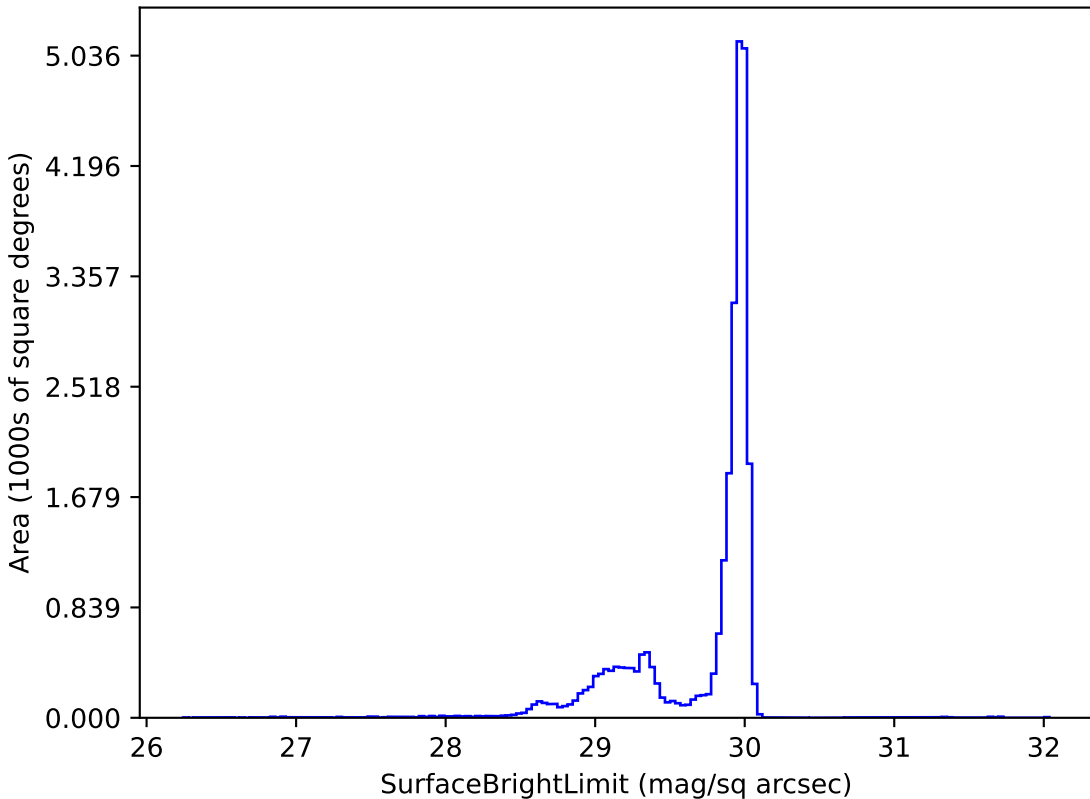
weather_cloudso10v3.4_10yrs i: SurfaceBrightLimit
