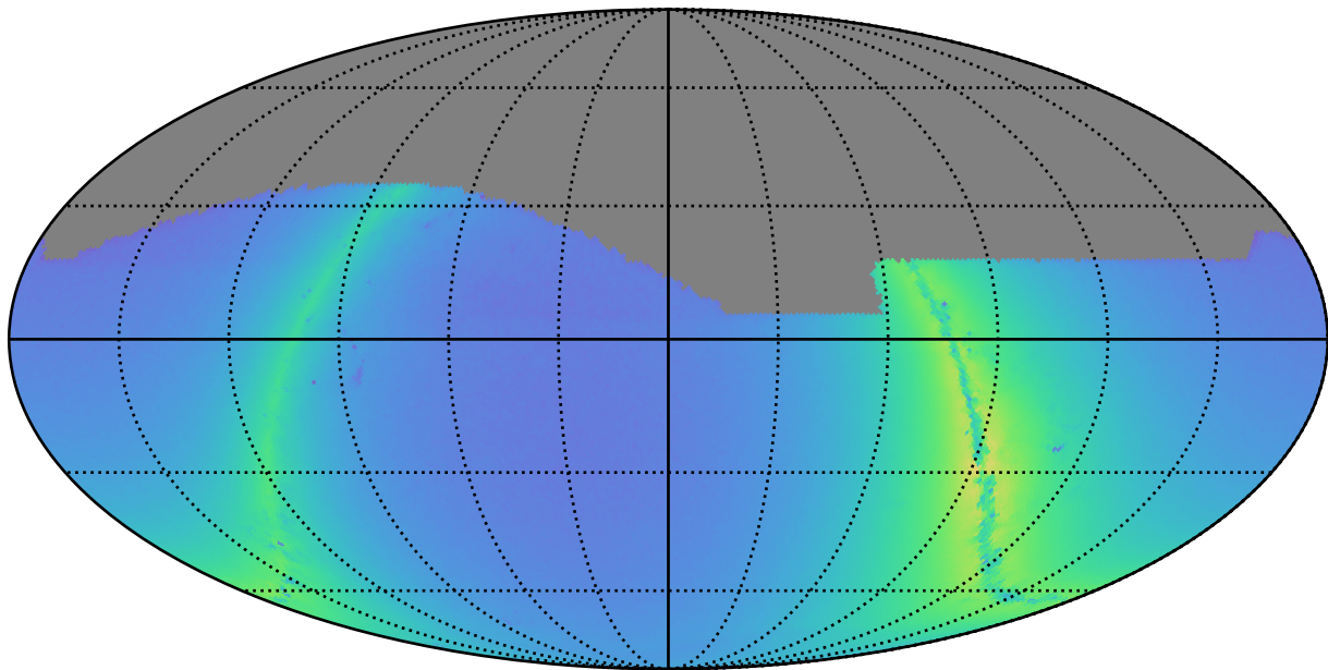
weather_cloudso10v3.4_10yrs z: Nstars_no_crowding
