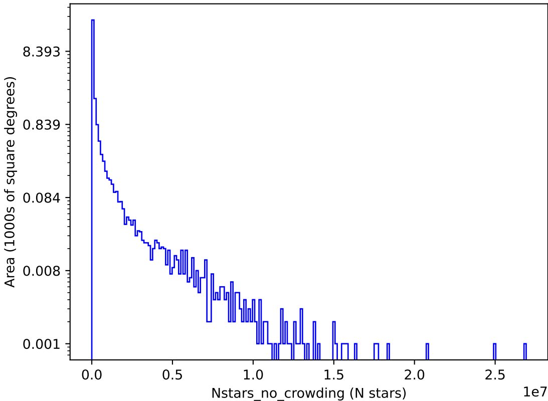
weather_cloudso10v3.4_10yrs z: Nstars_no_crowding
