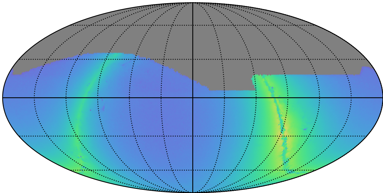
weather_cloudso10v3.4_10yrs i: Nstars_no_crowding
