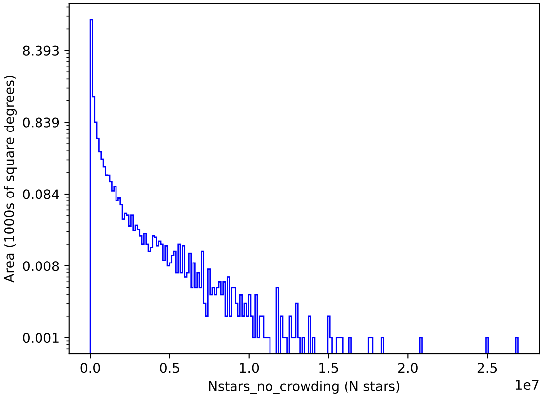
weather_cloudso10v3.4_10yrs i: Nstars_no_crowding
