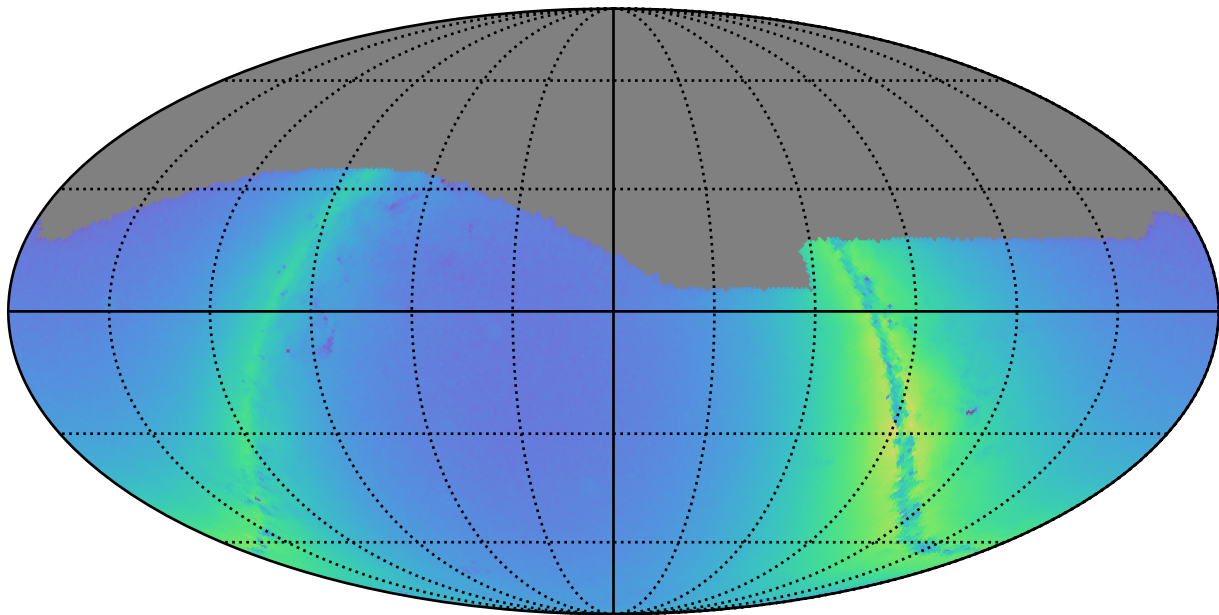
weather_cloudso10v3.4_10yrs g: Nstars_no_crowding
