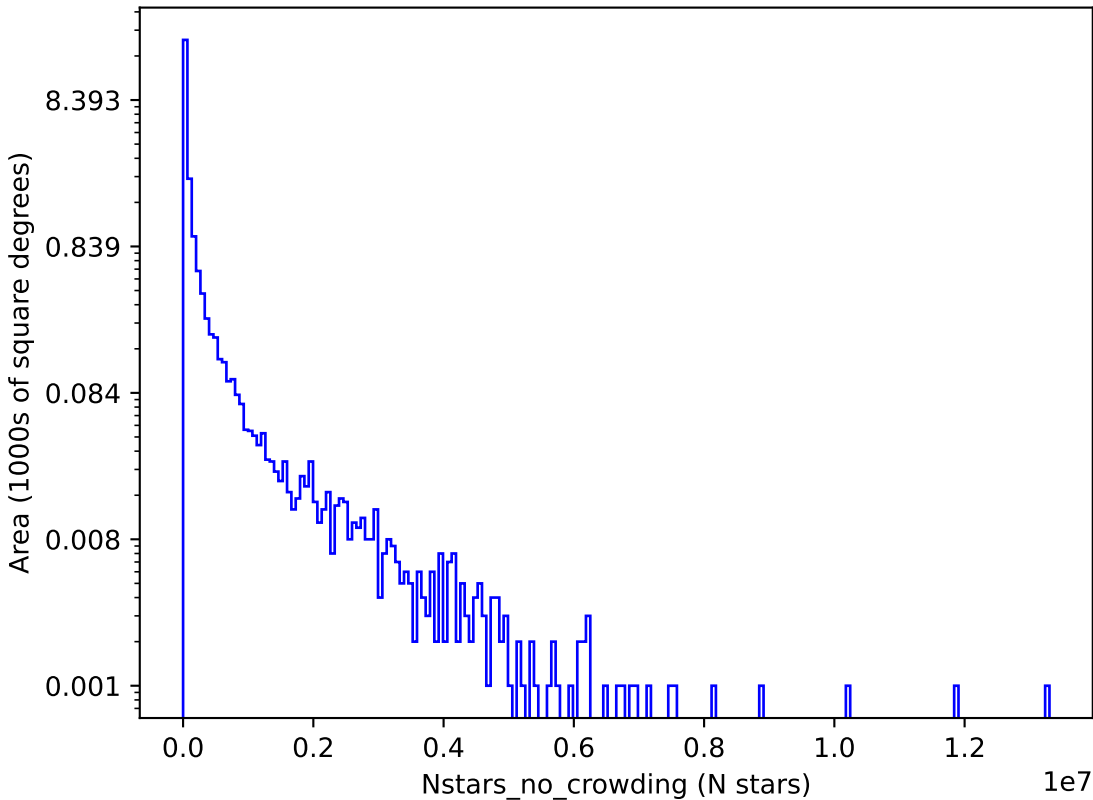
weather_cloudso10v3.4_10yrs g: Nstars_no_crowding
