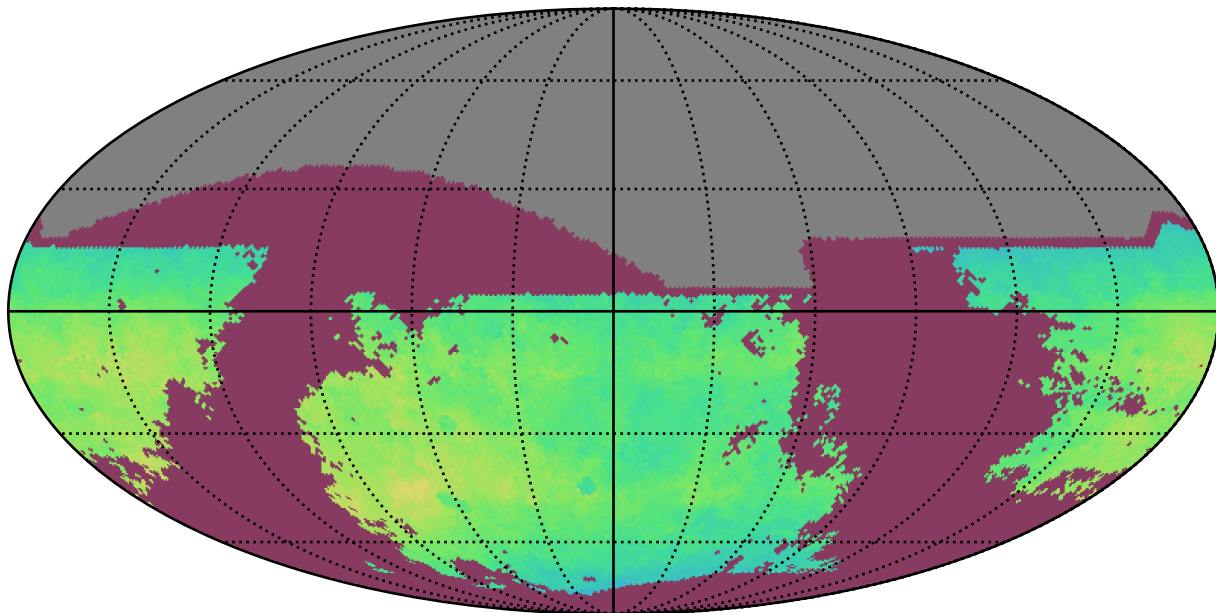
weather_cloudso10v3.4_10yrs i: NgalScale
