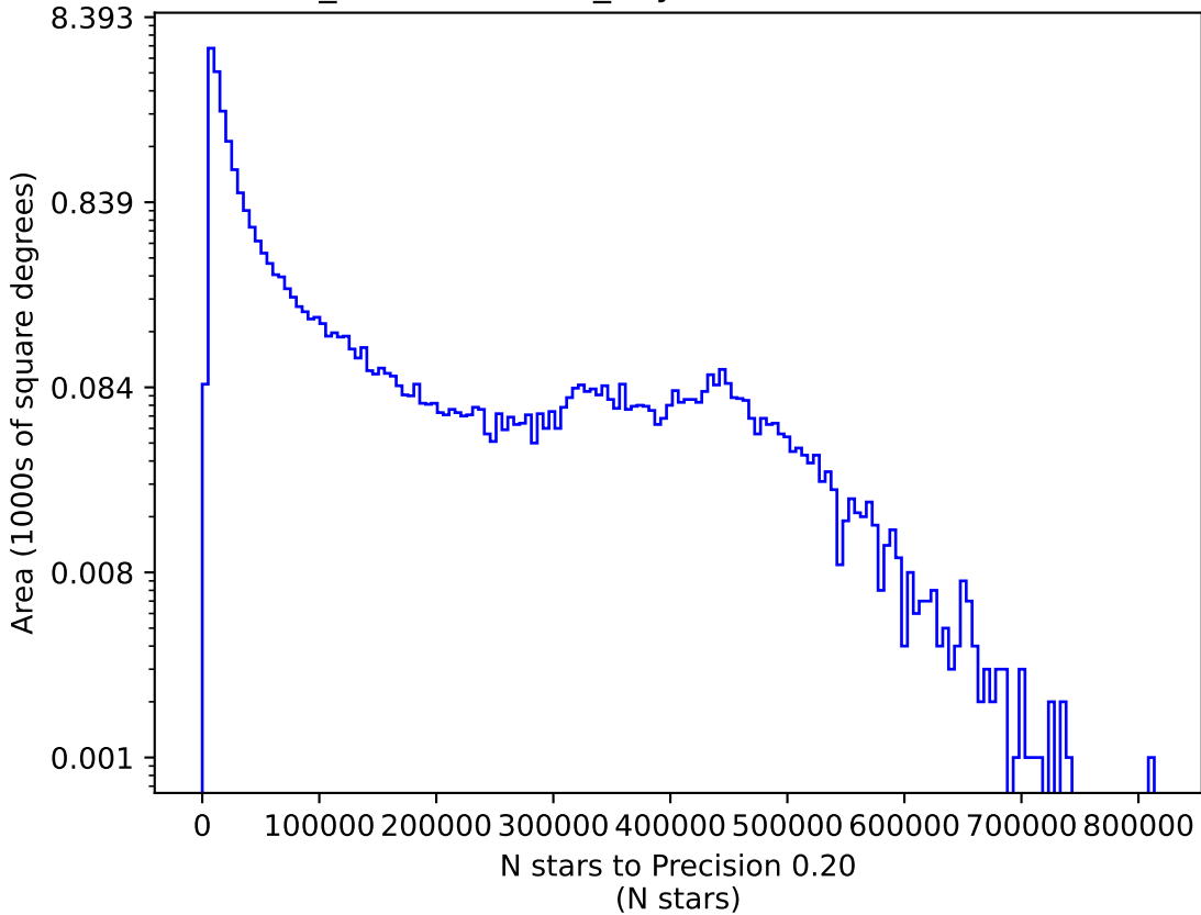
weather_cloudso10v3.4_10yrs i: N stars to Precision 0.20
