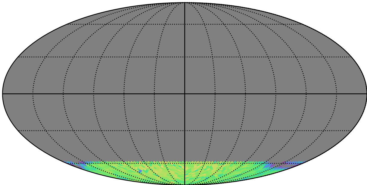
weather_cloudso10v3.4_10yrs gi SCP: LVDwarfs
