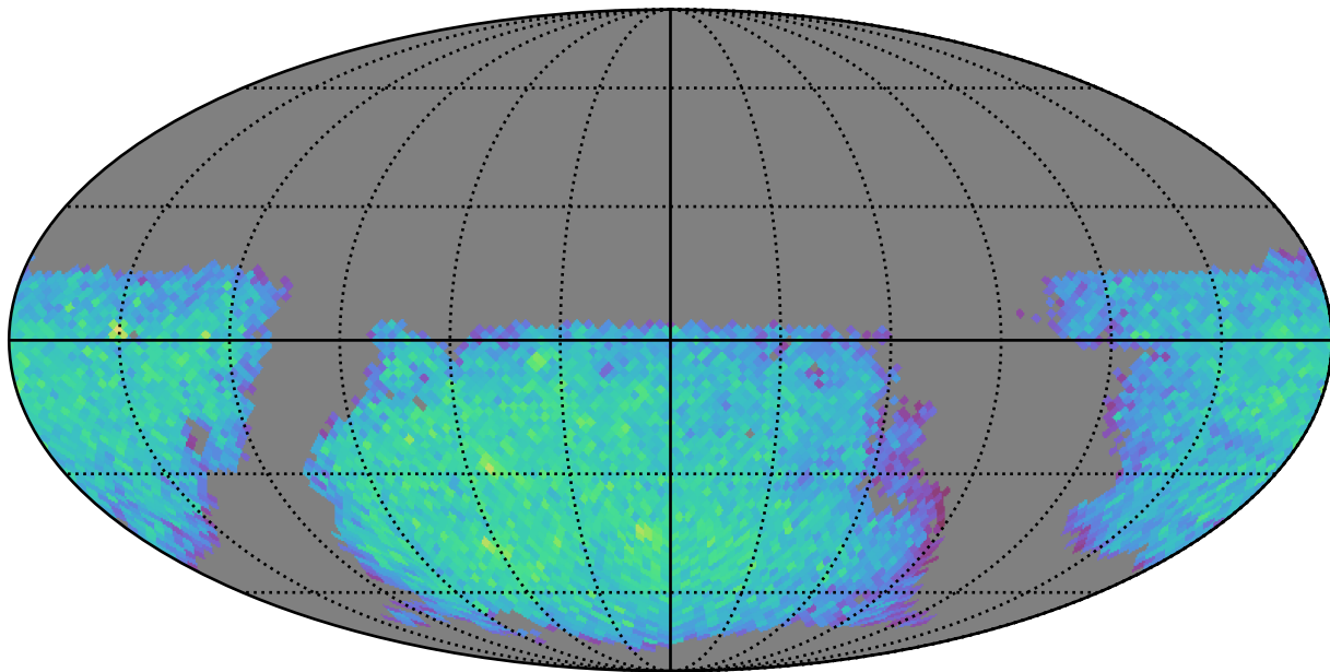
weather_cloudso10v3.4_10yrs gi: LVDwarfs
