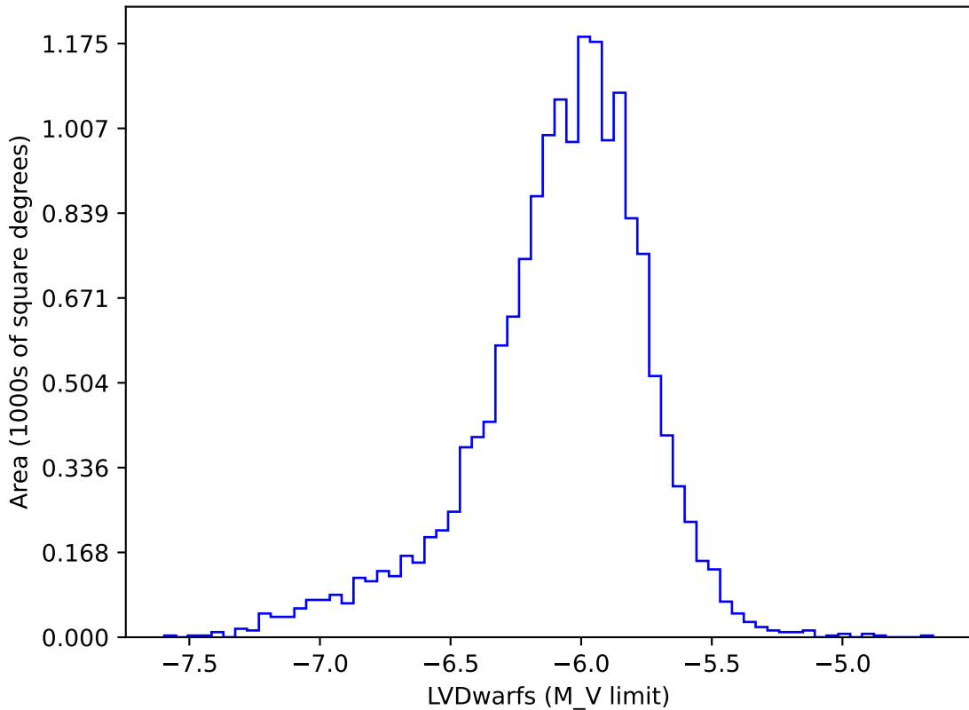
weather_cloudso10v3.4_10yrs gi: LVDwarfs
