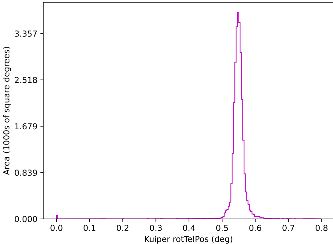
weather_cloudso10v3.4_10yrs z: Kuiper rotTelPos
