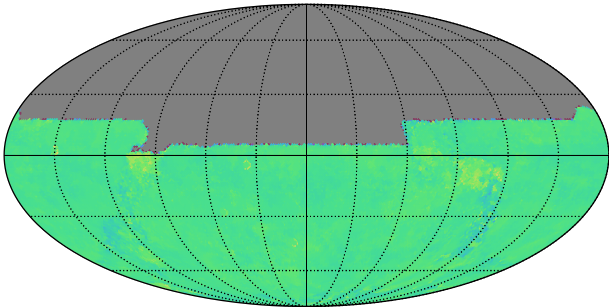
weather_cloudso10v3.4_10yrs u: Kuiper rotTelPos
