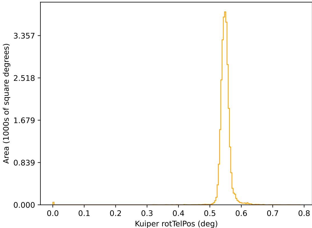
weather_cloudso10v3.4_10yrs r: Kuiper rotTelPos
