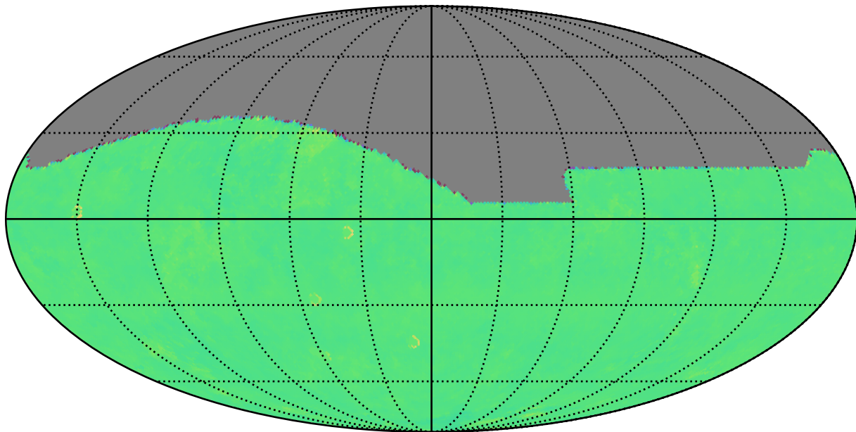
weather_cloudso10v3.4_10yrs i: Kuiper rotTelPos
