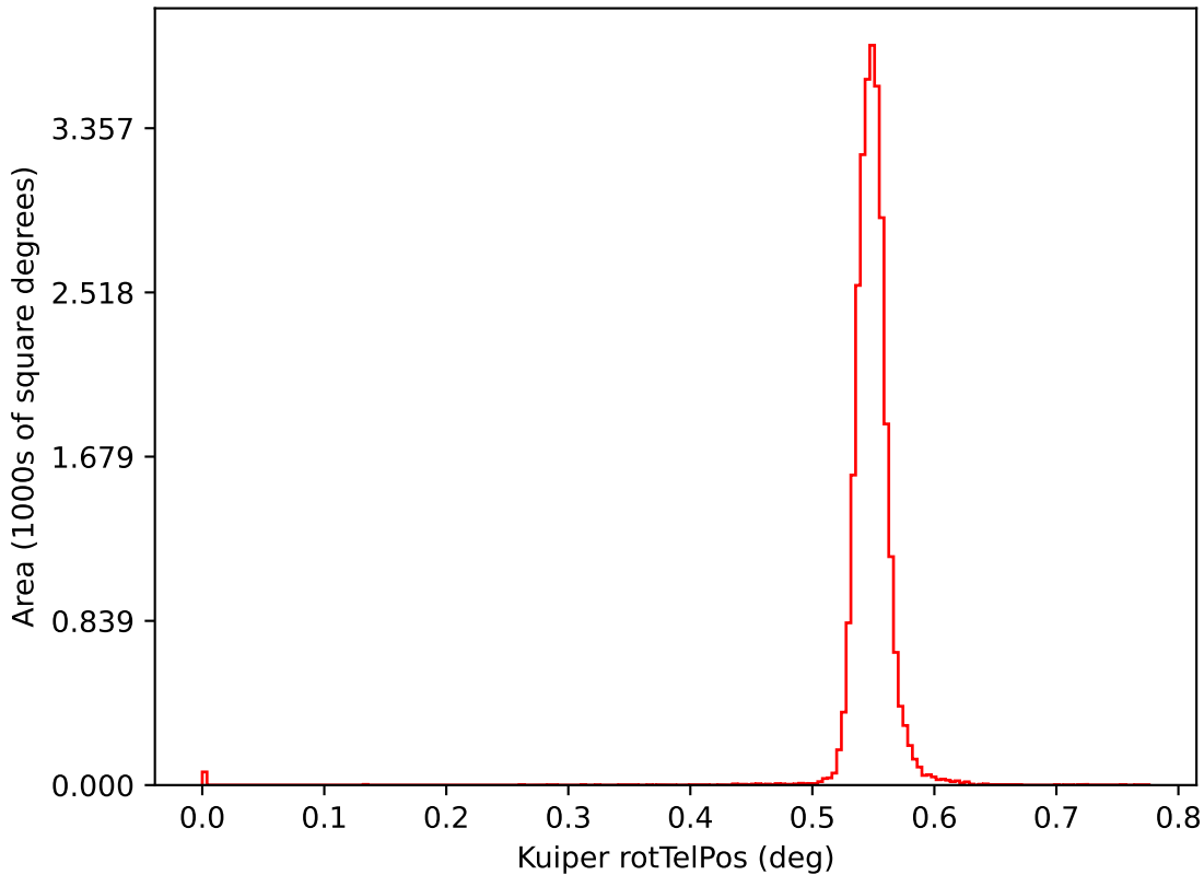
weather_cloudso10v3.4_10yrs i: Kuiper rotTelPos
