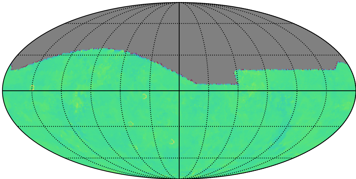
weather_cloudso10v3.4_10yrs g: Kuiper rotTelPos
