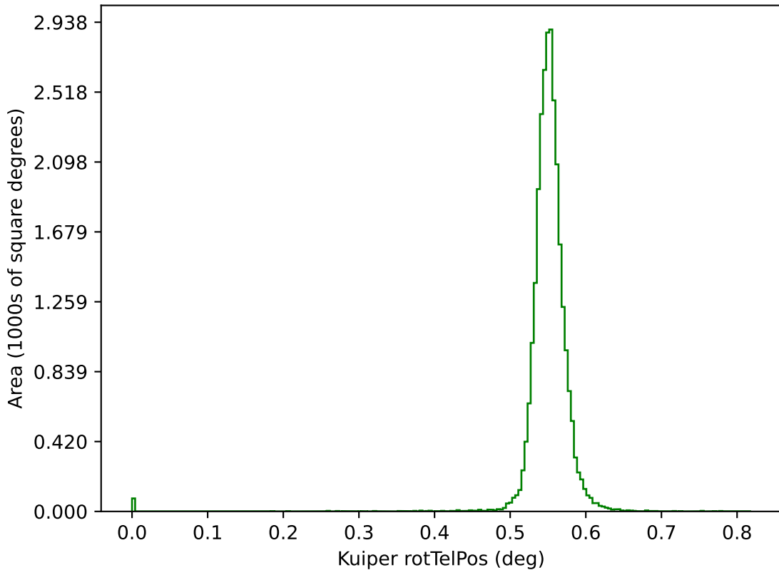
weather_cloudso10v3.4_10yrs g: Kuiper rotTelPos
