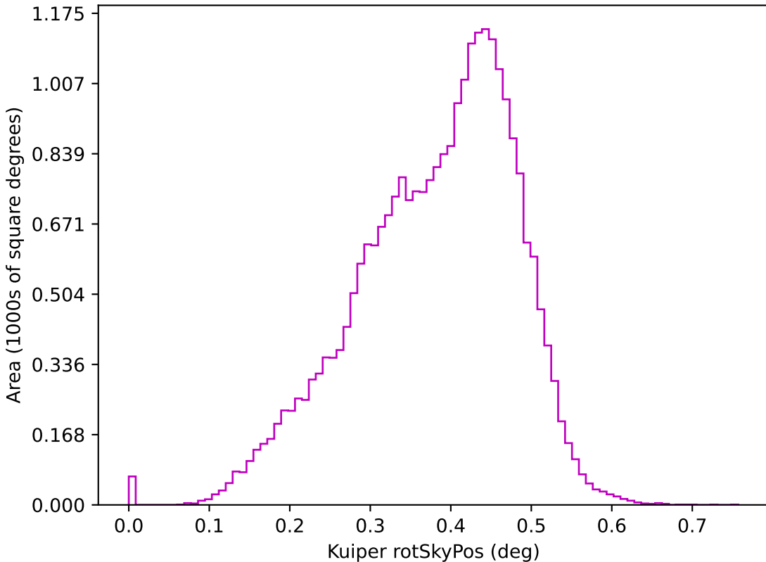
weather_cloudso10v3.4_10yrs z: Kuiper rotSkyPos
