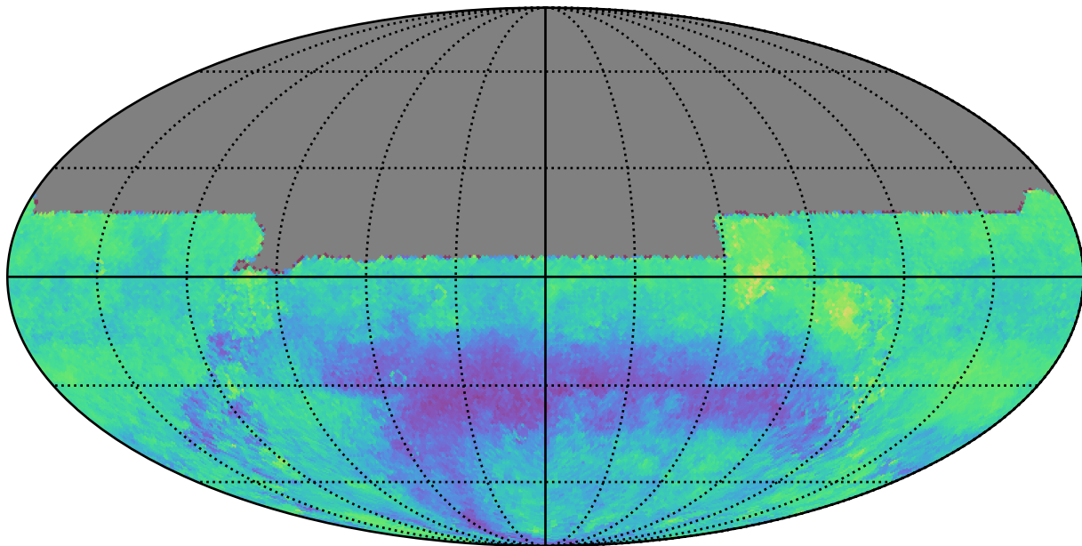
weather_cloudso10v3.4_10yrs u: Kuiper rotSkyPos
