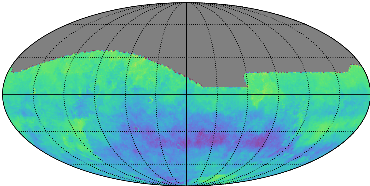
weather_cloudso10v3.4_10yrs i: Kuiper rotSkyPos
