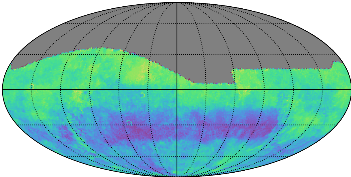
weather_cloudso10v3.4_10yrs g: Kuiper rotSkyPos
