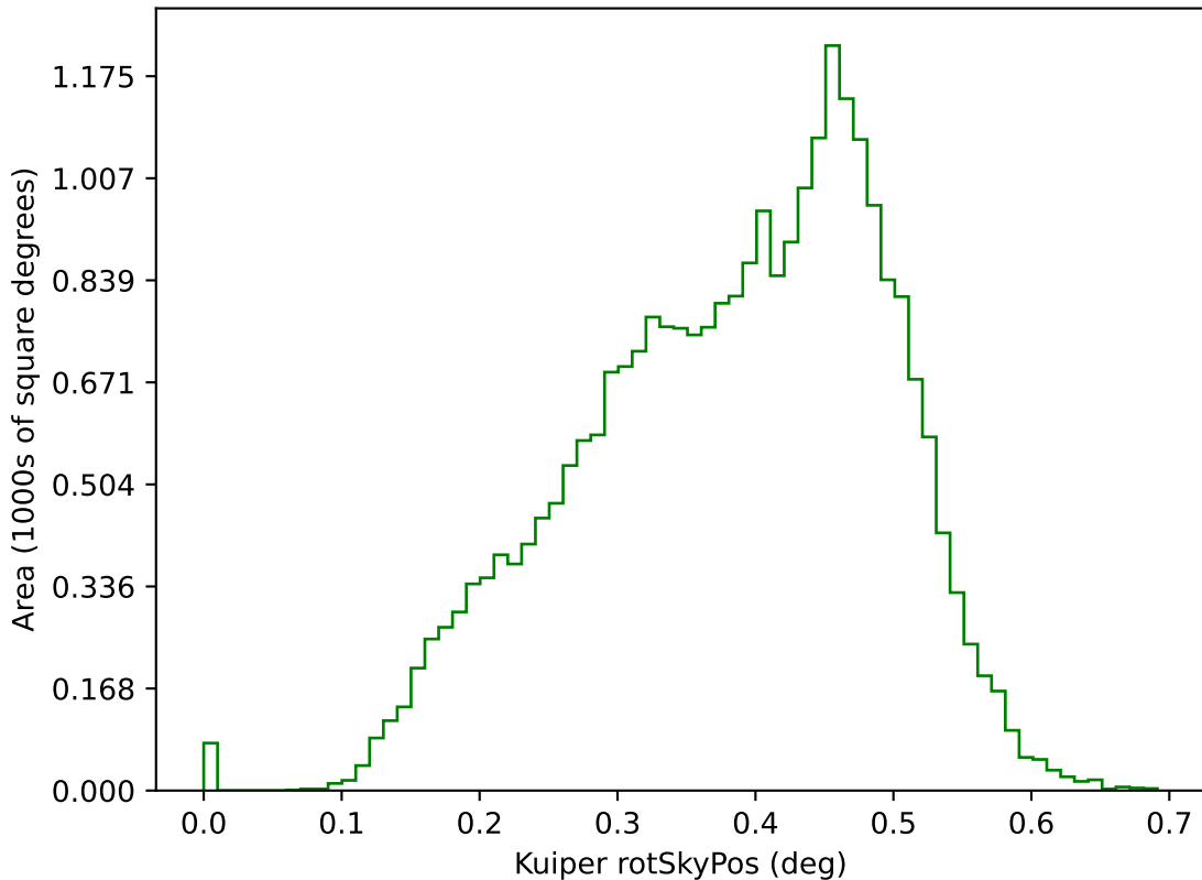
weather_cloudso10v3.4_10yrs g: Kuiper rotSkyPos
