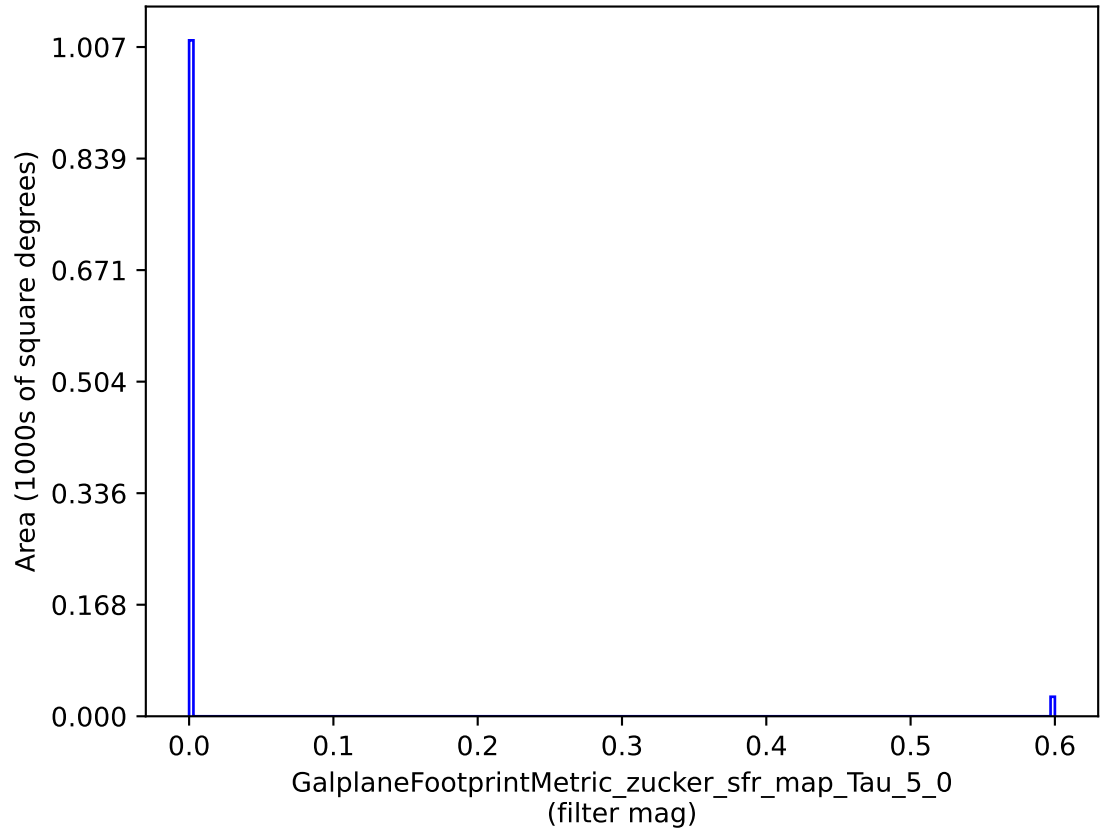
weather_cloudso10v3.4_10yrs : GalplaneFootprintMetric_zucker_sfr_map_Tau_5_0
