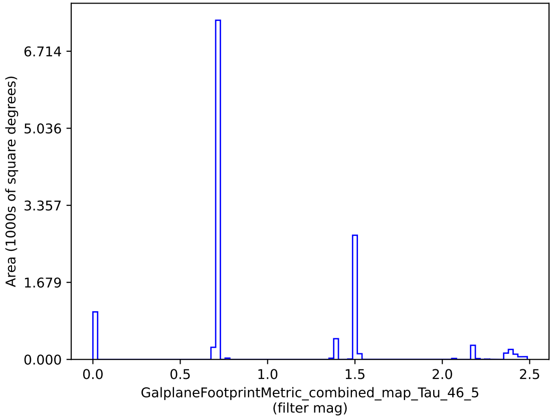
weather_cloudso10v3.4_10yrs : GalplaneFootprintMetric_combined_map_Tau_46_5
