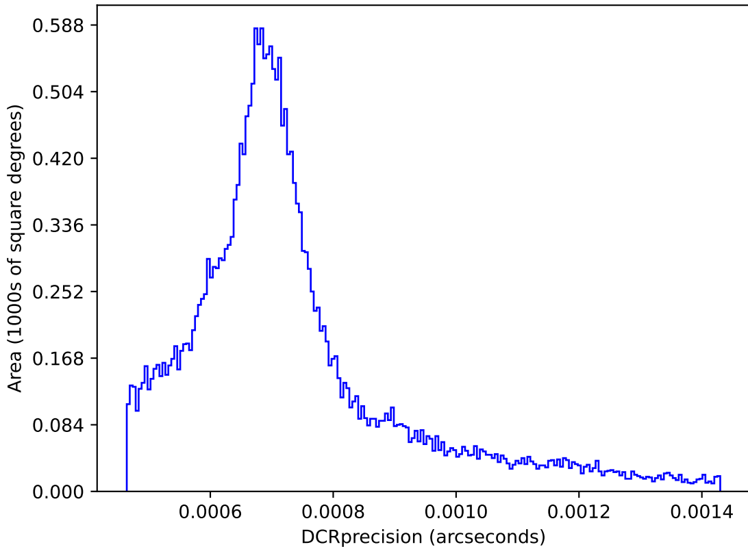
weather_cloudso10v3.4_10yrs : DCRprecision
