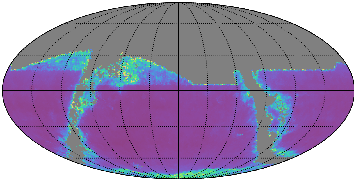
weather_cloudso10v3.4_10yrs z band: AGN SF_uncert
