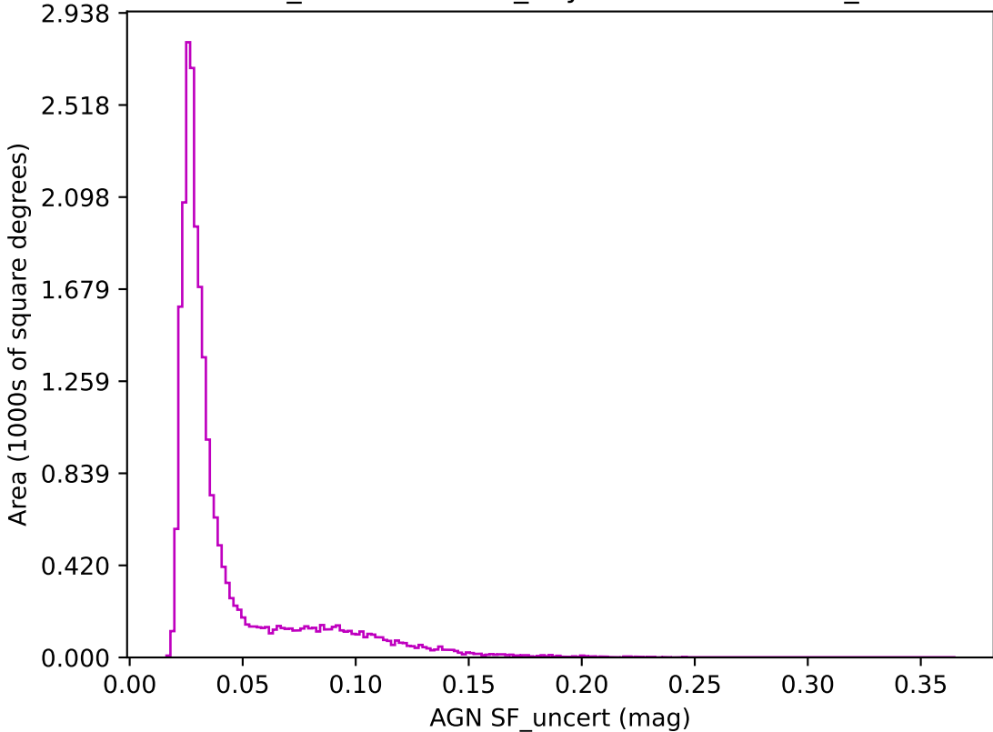
weather_cloudso10v3.4_10yrs z band: AGN SF_uncert
