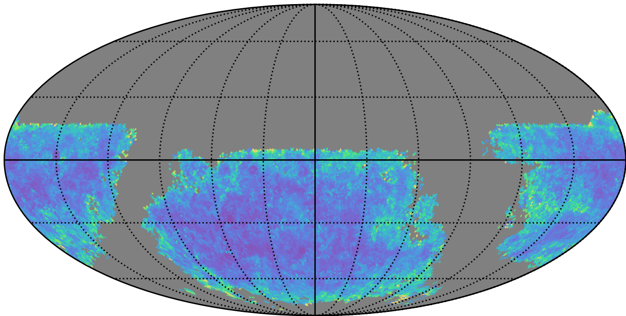
weather_cloudso10v3.4_10yrs u band: AGN SF_uncert
