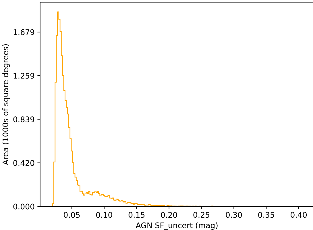
weather_cloudso10v3.4_10yrs r band: AGN SF_uncert
