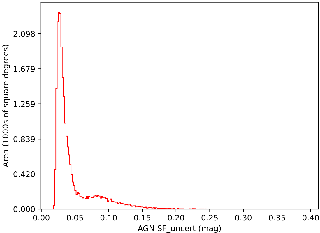
weather_cloudso10v3.4_10yrs i band: AGN SF_uncert
