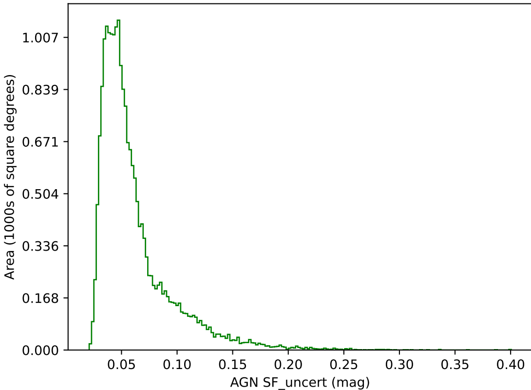
weather_cloudso10v3.4_10yrs g band: AGN SF_uncert
