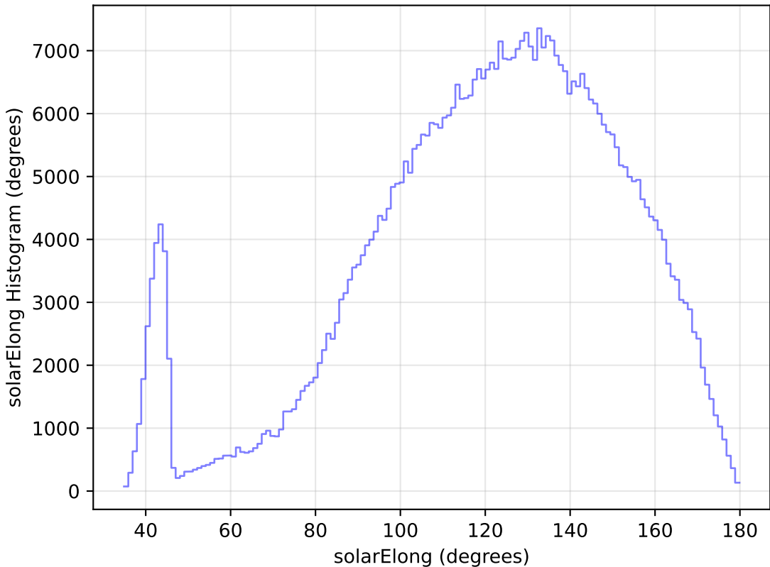
weather_cloudso10v3.4_10yrs WFD i band: solarElong Histogram
