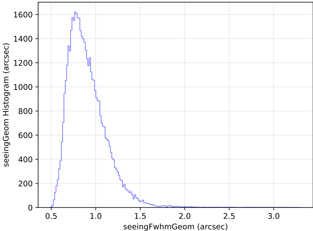
weather_cloudso10v3.4_10yrs Yr 1 y band: seeingGeom Histogram
