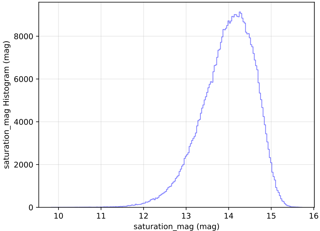
weather_cloudso10v3.4_10yrs WFD z band: saturation_mag Histogram
