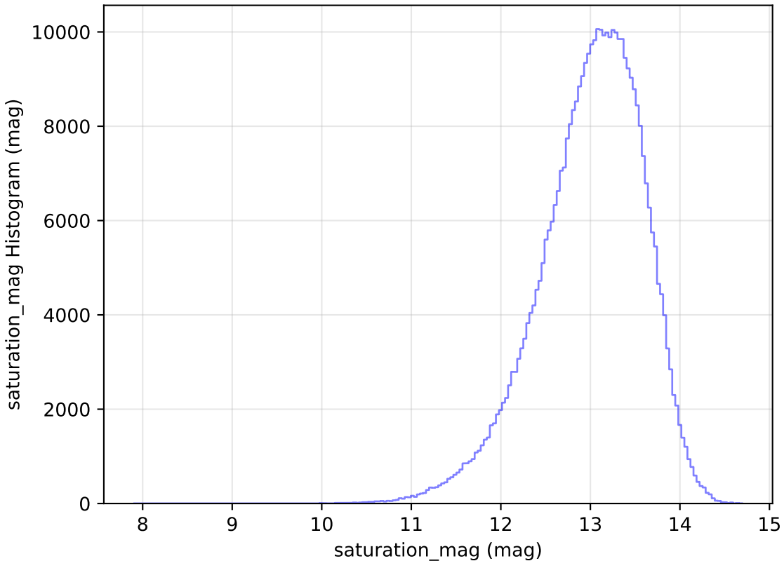
weather_cloudso10v3.4_10yrs WFD y band: saturation_mag Histogram
