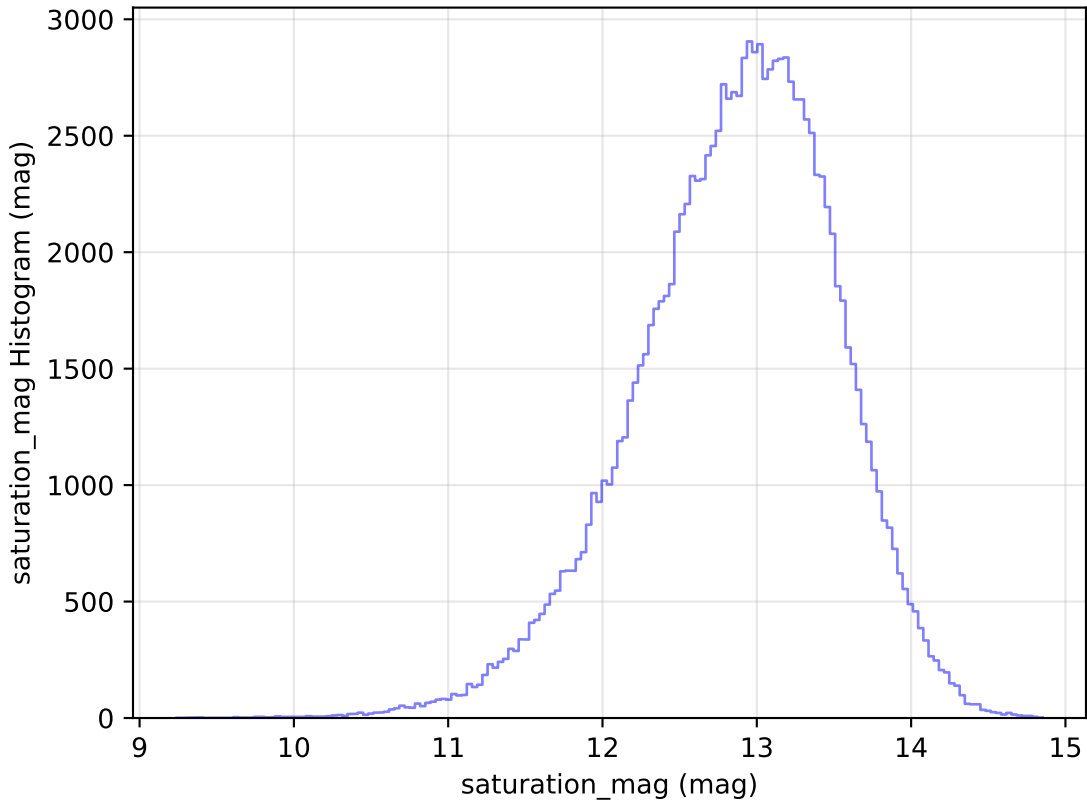
weather_cloudso10v3.4_10yrs WFD u band: saturation_mag Histogram
