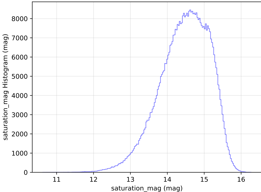
weather_cloudso10v3.4_10yrs WFD r band: saturation_mag Histogram
