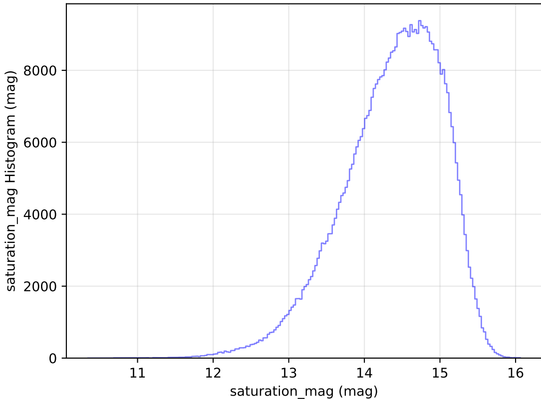
weather_cloudso10v3.4_10yrs WFD i band: saturation_mag Histogram
