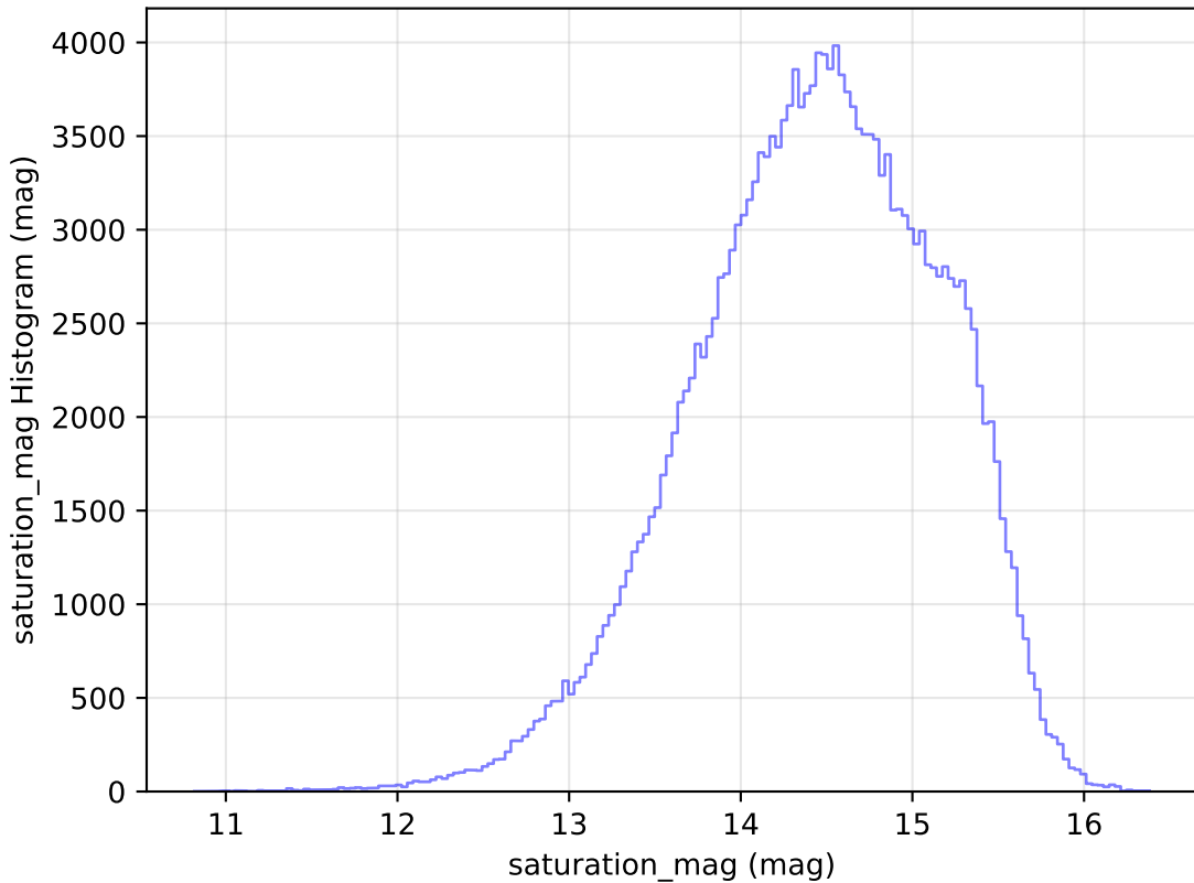
weather_cloudso10v3.4_10yrs WFD g band: saturation_mag Histogram
