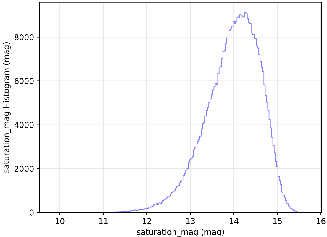
weather_cloudso10v3.4_10yrs All sky z band: saturation_mag Histogram
