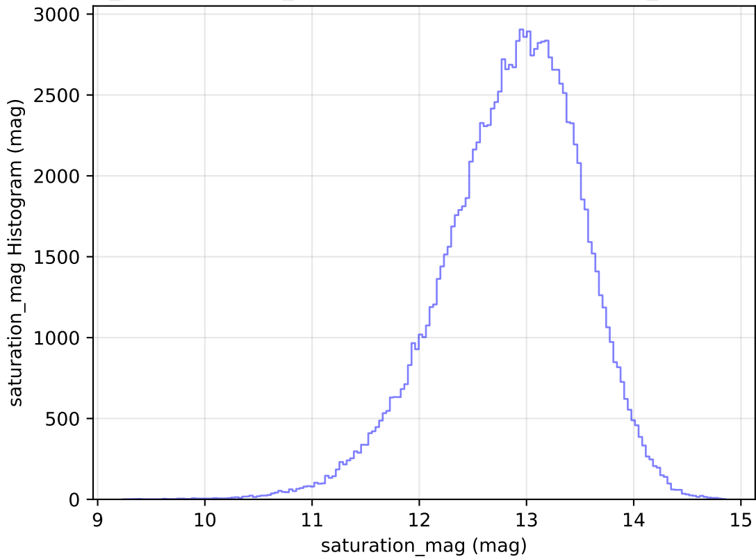
weather_cloudso10v3.4_10yrs All sky u band: saturation_mag Histogram
