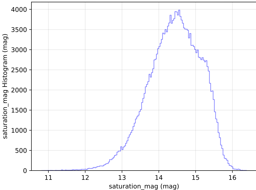
weather_cloudso10v3.4_10yrs All sky g band: saturation_mag Histogram
