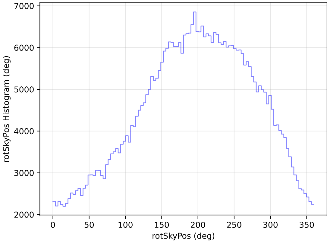
weather_cloudso10v3.4_10yrs WFD z band: rotSkyPos Histogram
