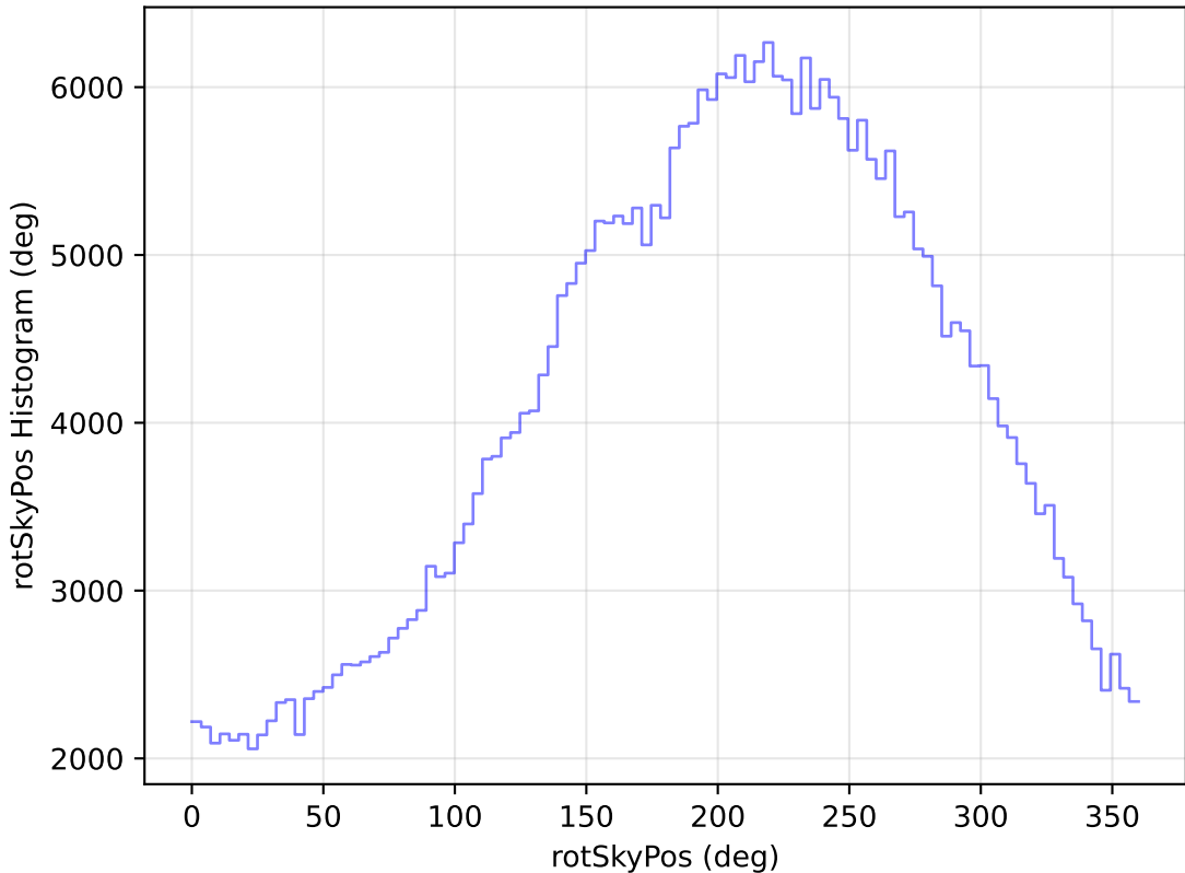
weather_cloudso10v3.4_10yrs WFD y band: rotSkyPos Histogram
