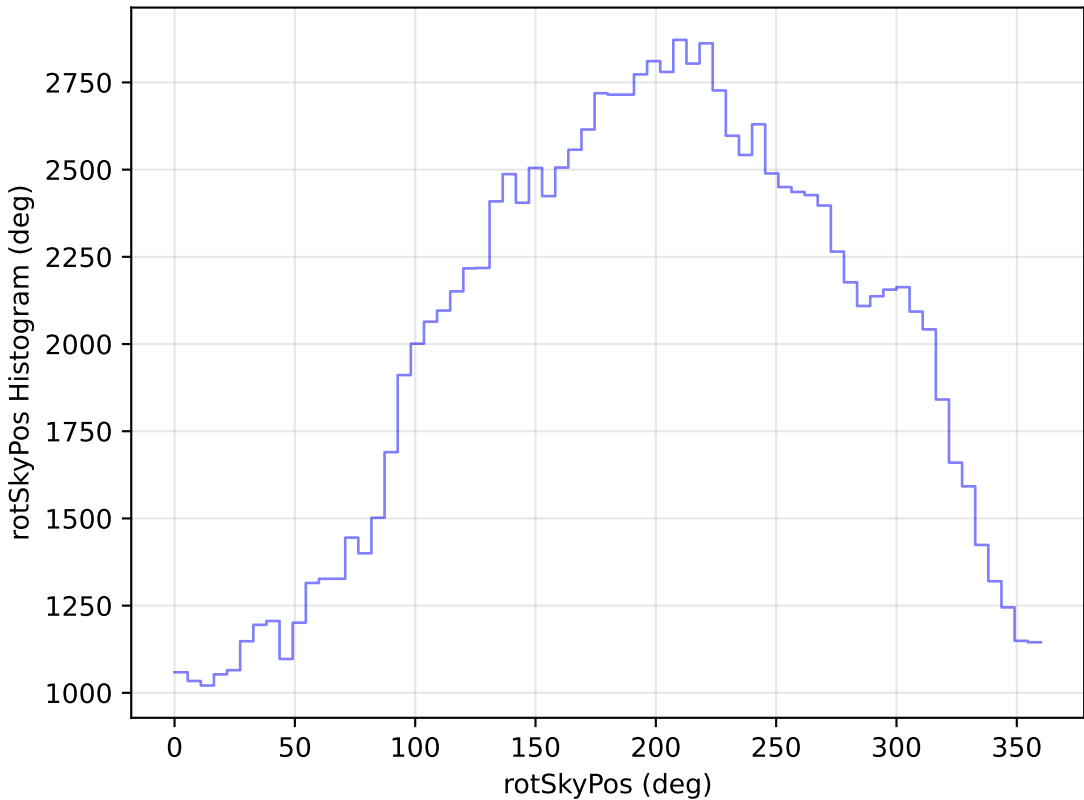
weather_cloudso10v3.4_10yrs WFD u band: rotSkyPos Histogram
