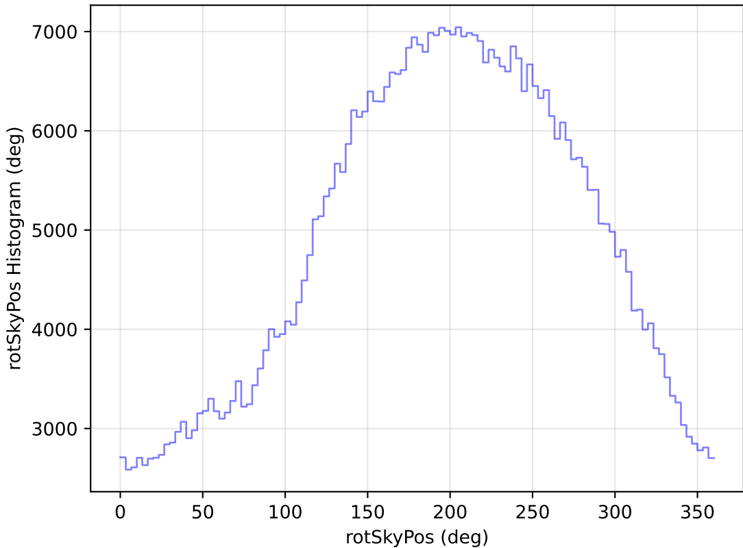
weather_cloudso10v3.4_10yrs WFD i band: rotSkyPos Histogram
