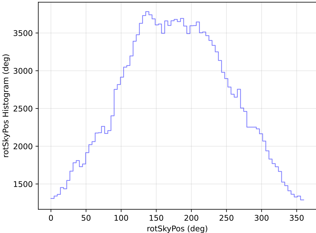
weather_cloudso10v3.4_10yrs WFD g band: rotSkyPos Histogram
